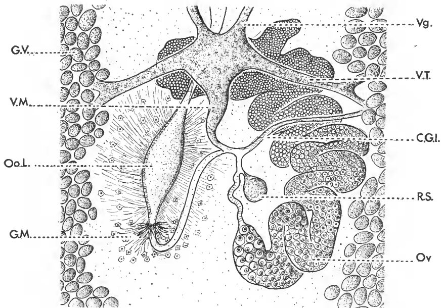
FIG. 4. — Détail de l'anatomie du genre Epicotyle n. g. C.G.I., canal génito-intestinal; G.M., glandes de Mehlis; G.V., glandes vitellogènes; Oo.L., ootype lisse; Ov., ovaire; R.S., réceptacle séminal; Vg., vagin; V.M., vitelloducte médian; V.T., vitelloducte transverse.
